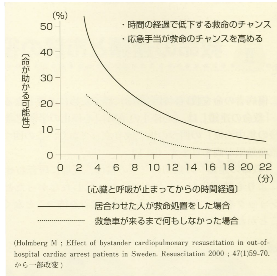
図1 救命曲線
