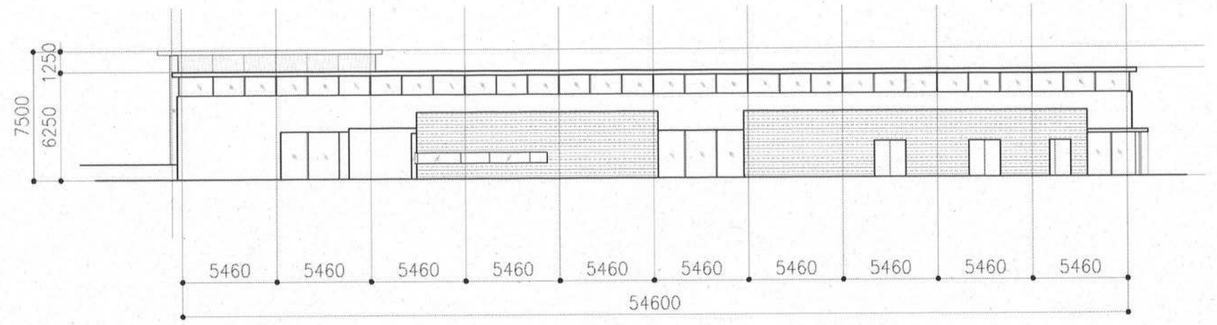
西立面图
