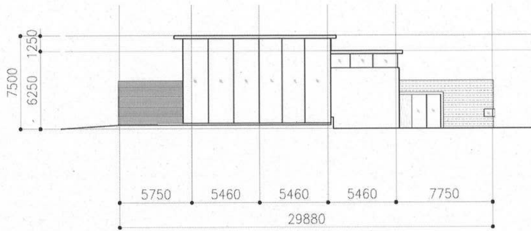
北立面图
