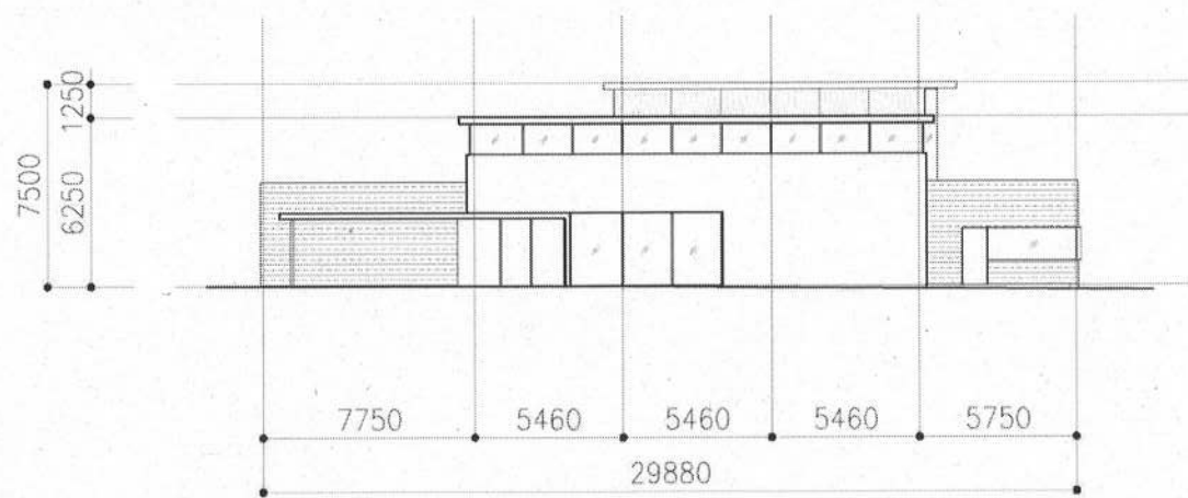
南立面图
