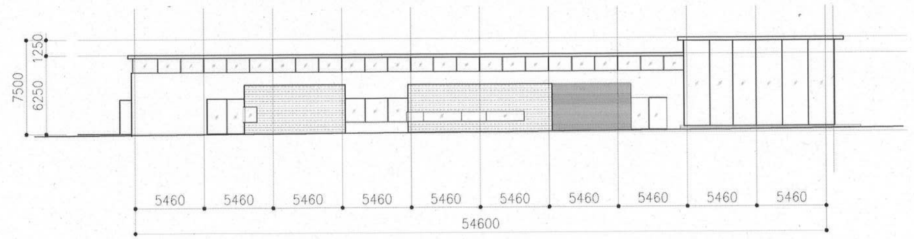
東立面图
